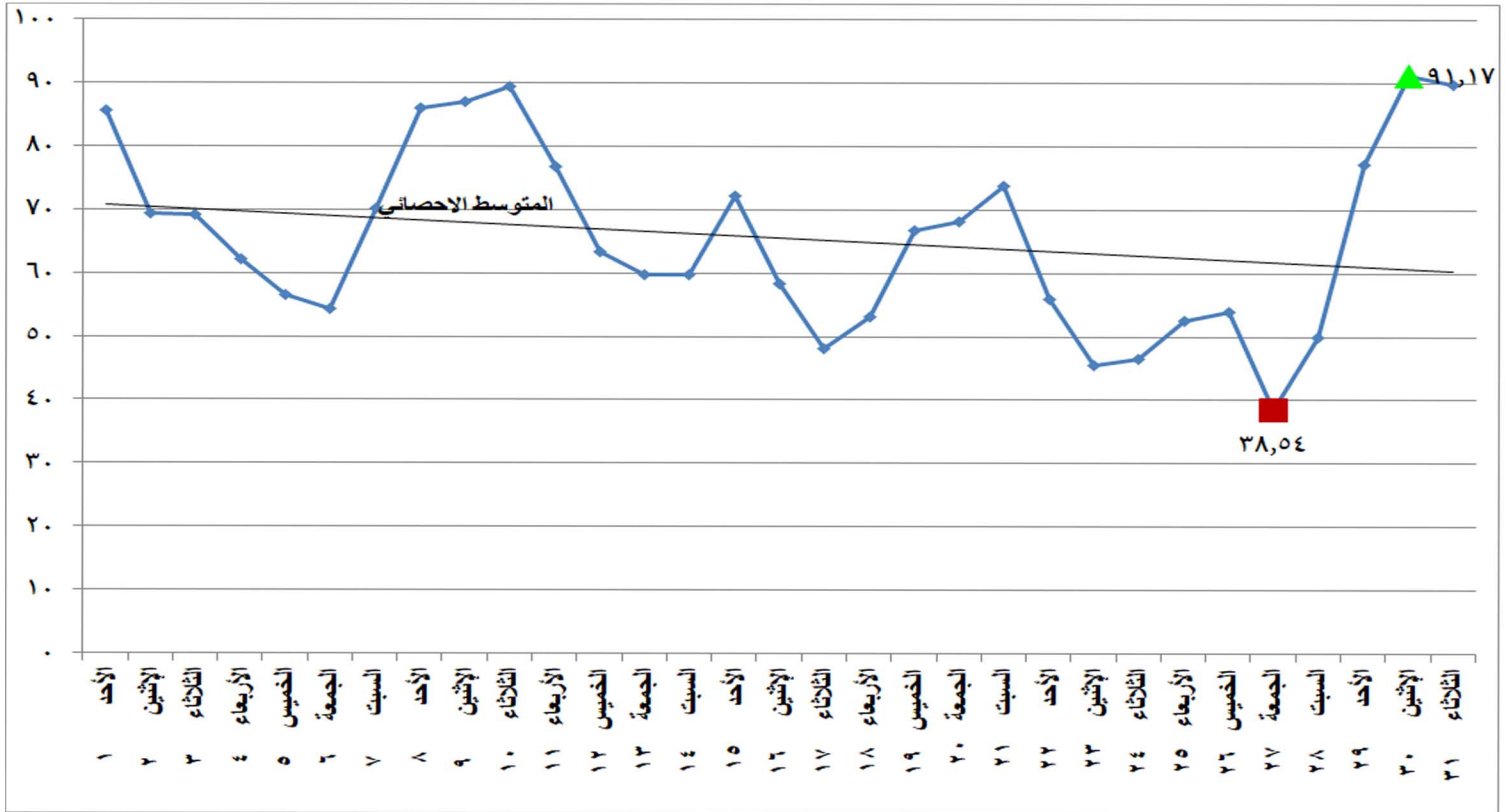
شكل (١٩) الطاقة الكهربائية المنتجة من المازوت خلال شهر مايو ٢٠٢٢
