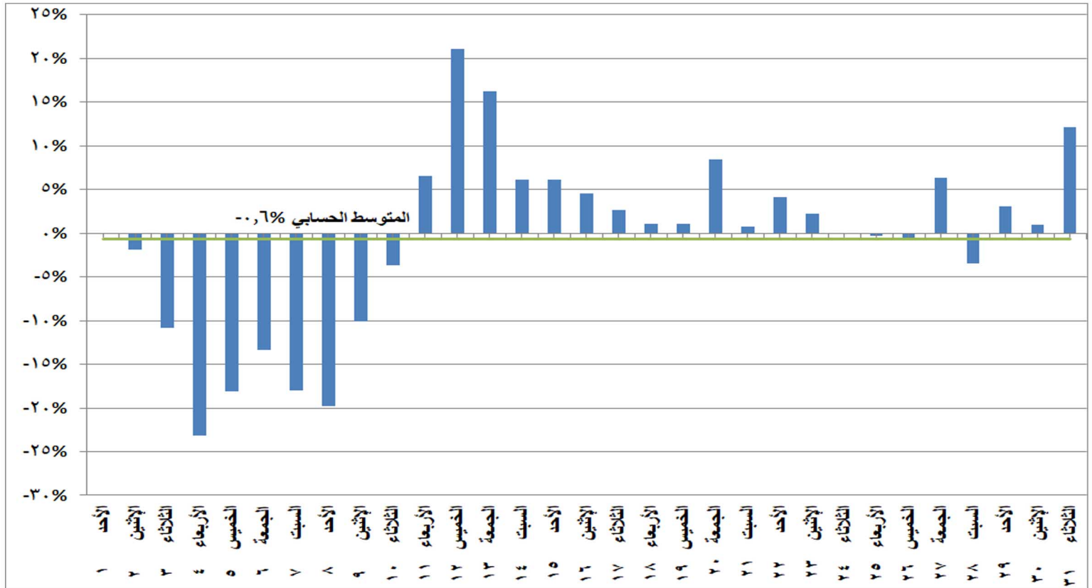
شكل (٩) النسب المئوية للتغير في الحمل الاقصى خلال شهر مايو ٢٠٢٢ مقارنة باليوم المماثل من العام الماضي
