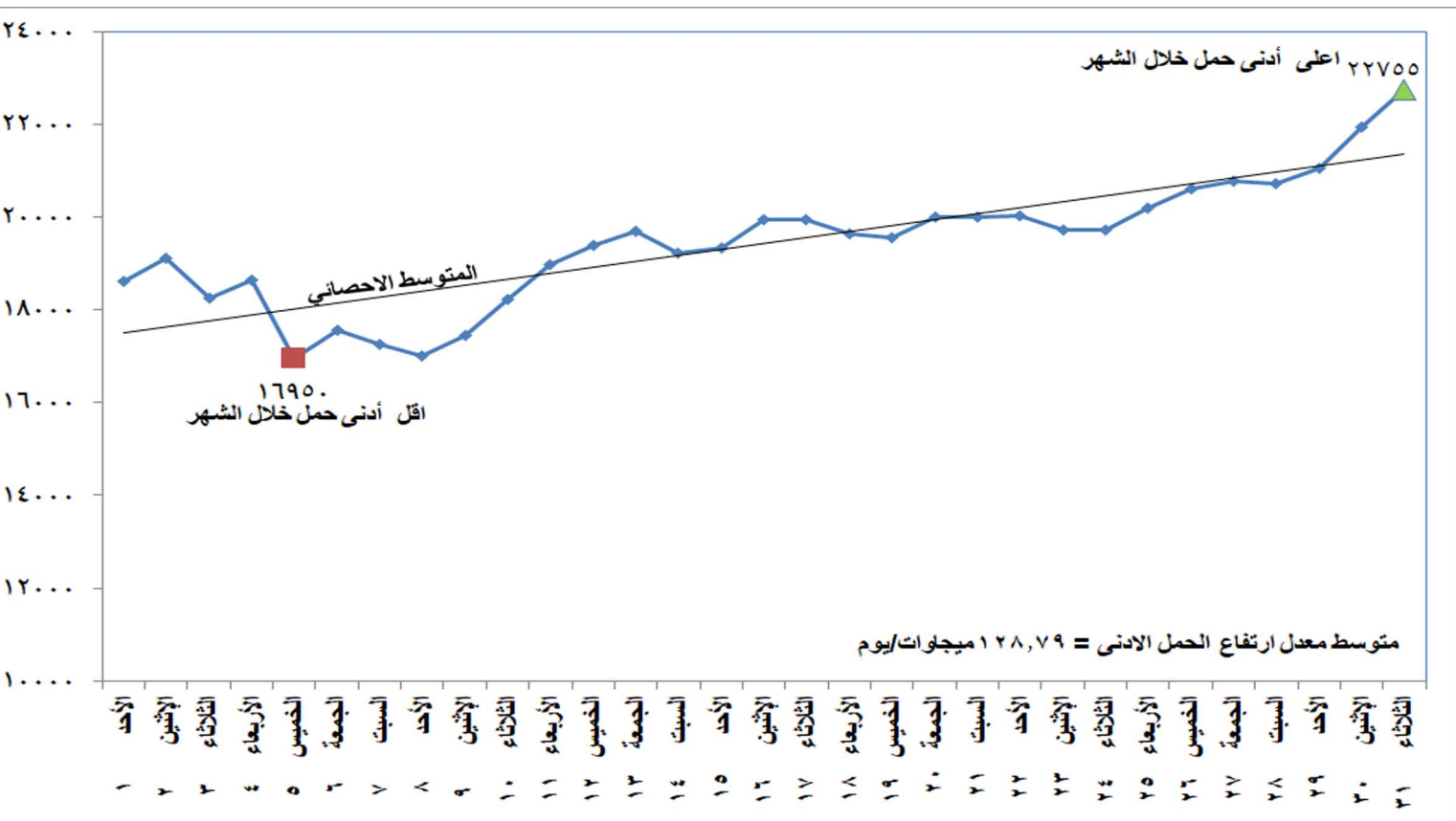
شكل (٢) تطور الحمل الأدنى اليومي خلال شهر مايو ٢٠٢٢
