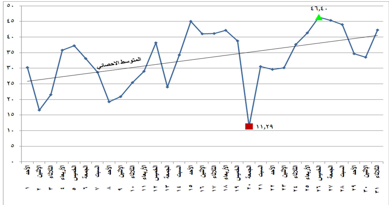
شكل (٢٥) الطاقة الكهربائية المنتجة من الرياح والشمس خلال شهر مايو ٢٠٢٢
