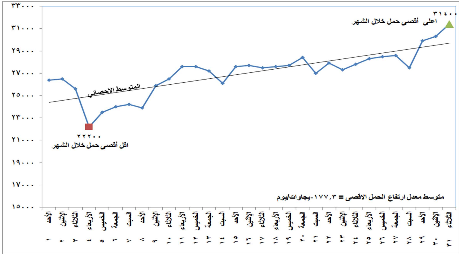
شكل (١) تطور الحمل الاقصى اليومي خلال شهر مايو ٢٠٢٢
