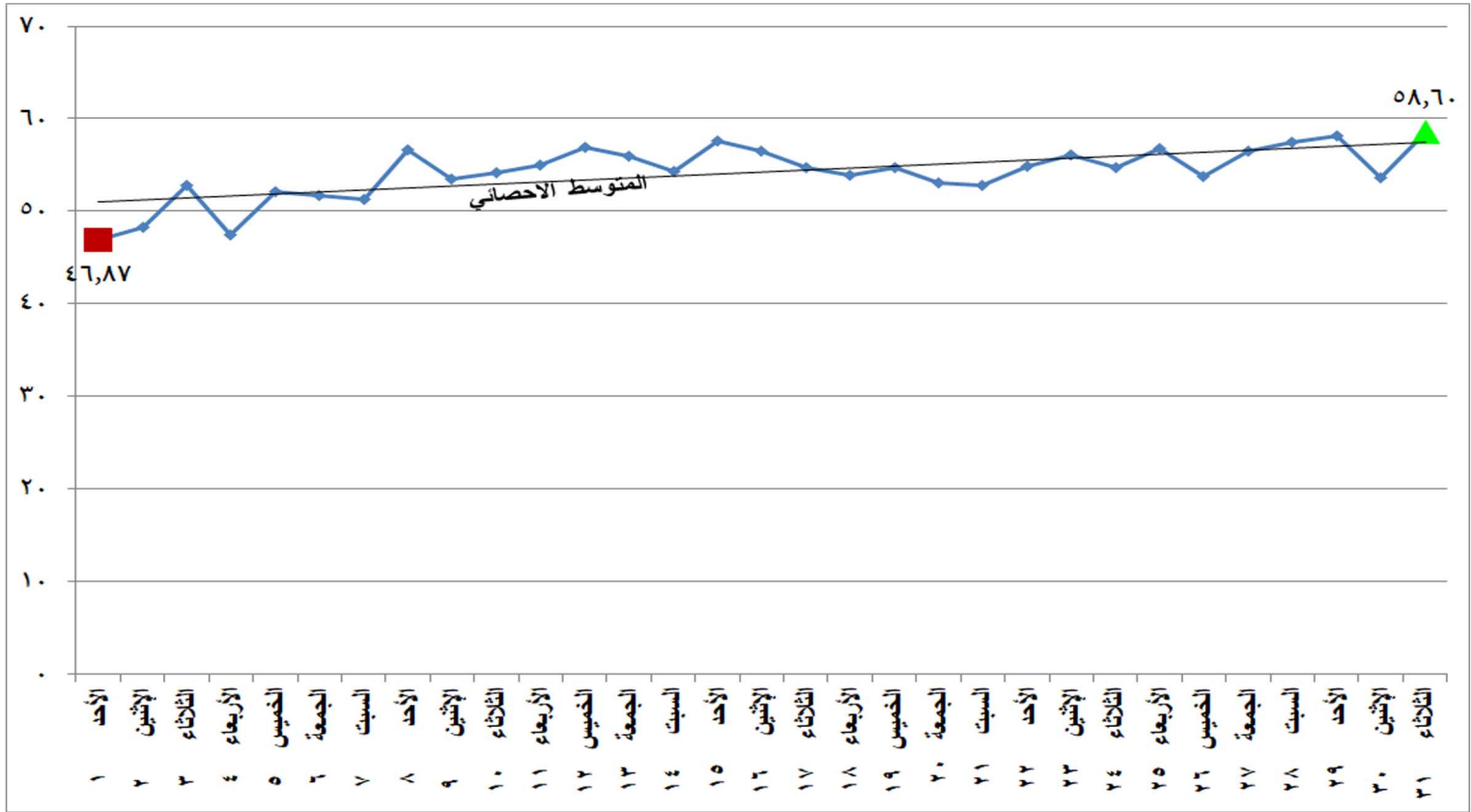
شكل (٢٣) الطاقة الكهربائية المنتجة من المصادر المائية خلال شهر مايو ٢٠٢٢
