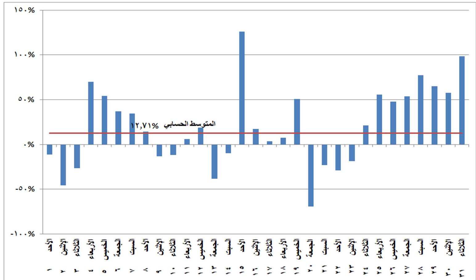
شكل (٢٦) نسب التغير في استخدام الرياح والشمس في إنتاج الطاقة الكهربائية خلال شهر مايو ٢٠٢٢ مقارنة بالشهر المماثل من العام السابق
