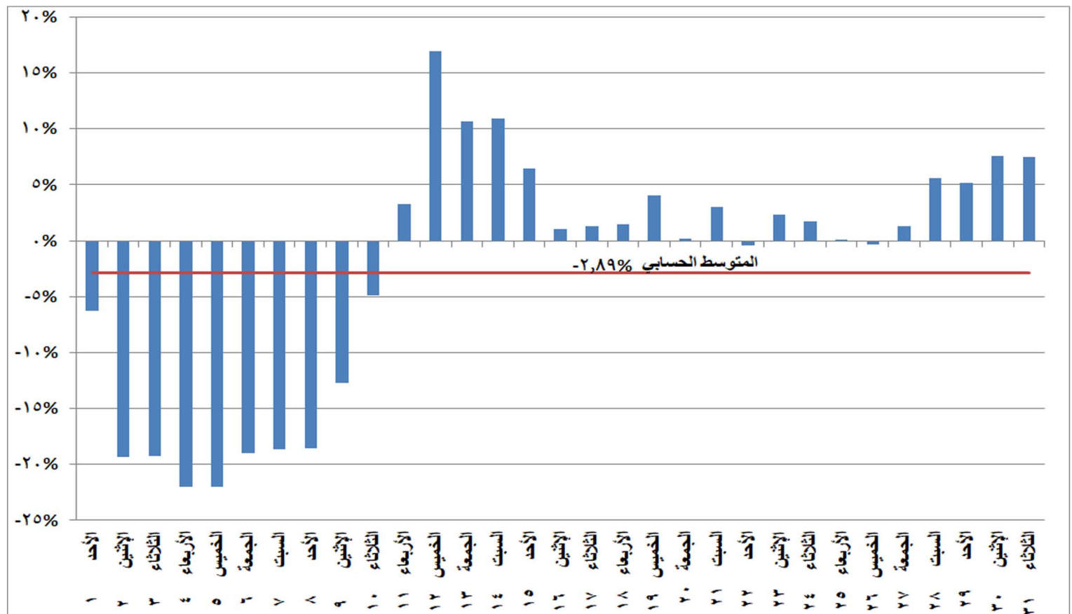
شكل (١٦) نسب التغير في الطاقة الكهربائية المنتجة خلال شهر مايو ٢٠٢٢ مقارنة بالشهر المماثل من العام السابق
