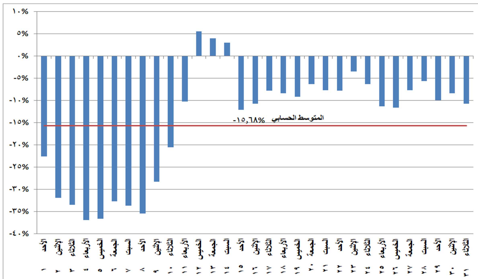
شكل (١٨) نسب التغير في استخدام الغاز الطبيعي في إنتاج الطاقة الكهربائية خلال شهر مايو ٢٠٢٢ مقارنة بالشهر المماثل من العام السابق
