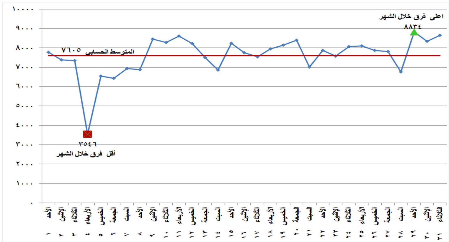
شكل (٣) الفرق بين أقصى وأدنى حمل خلال شهر مايو ٢٠٢٢
