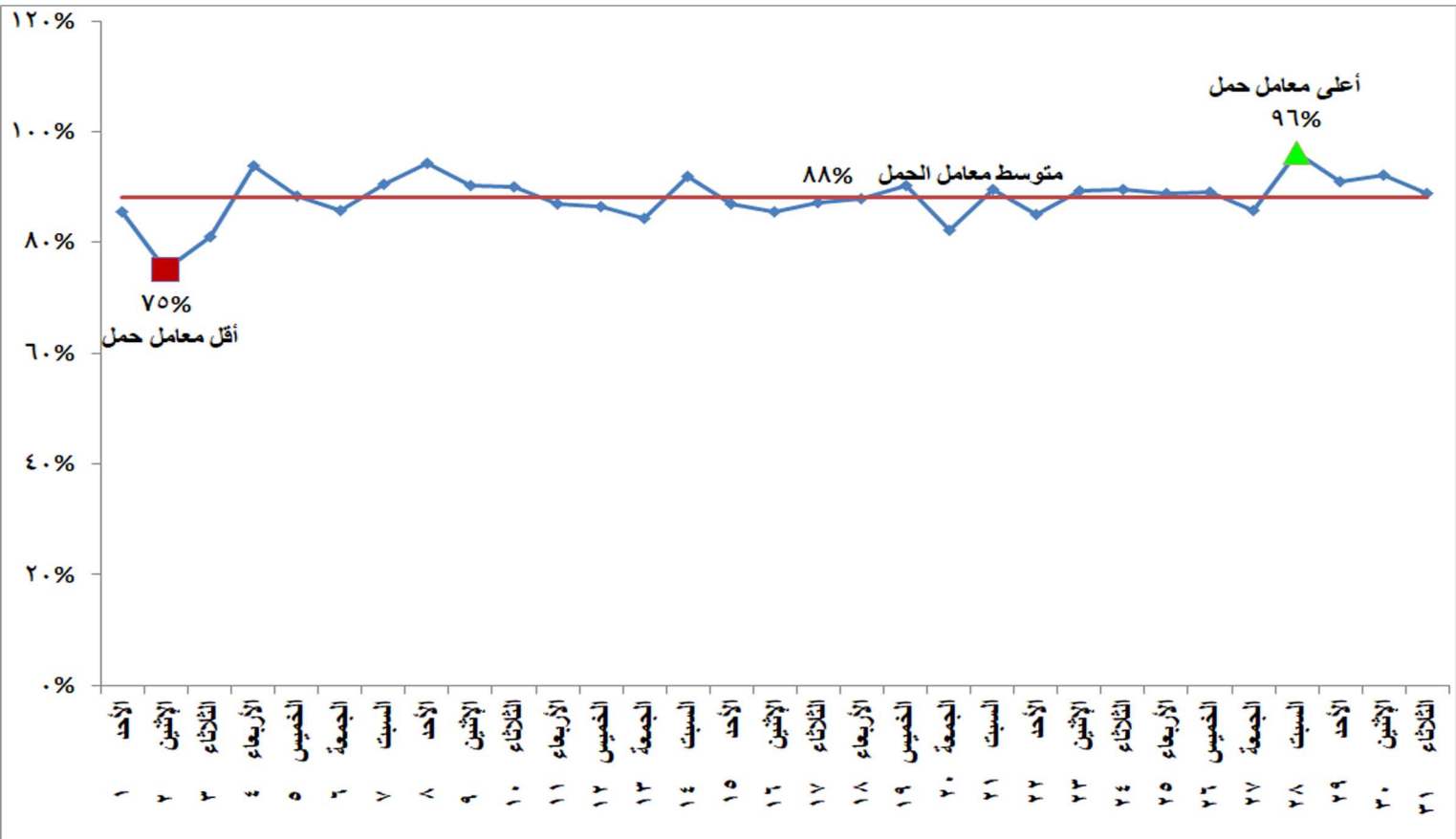
شكل (١٢) إجمالي معامل الحمل لوحدات الانتاج خلال شهر مايو ٢٠٢٢
