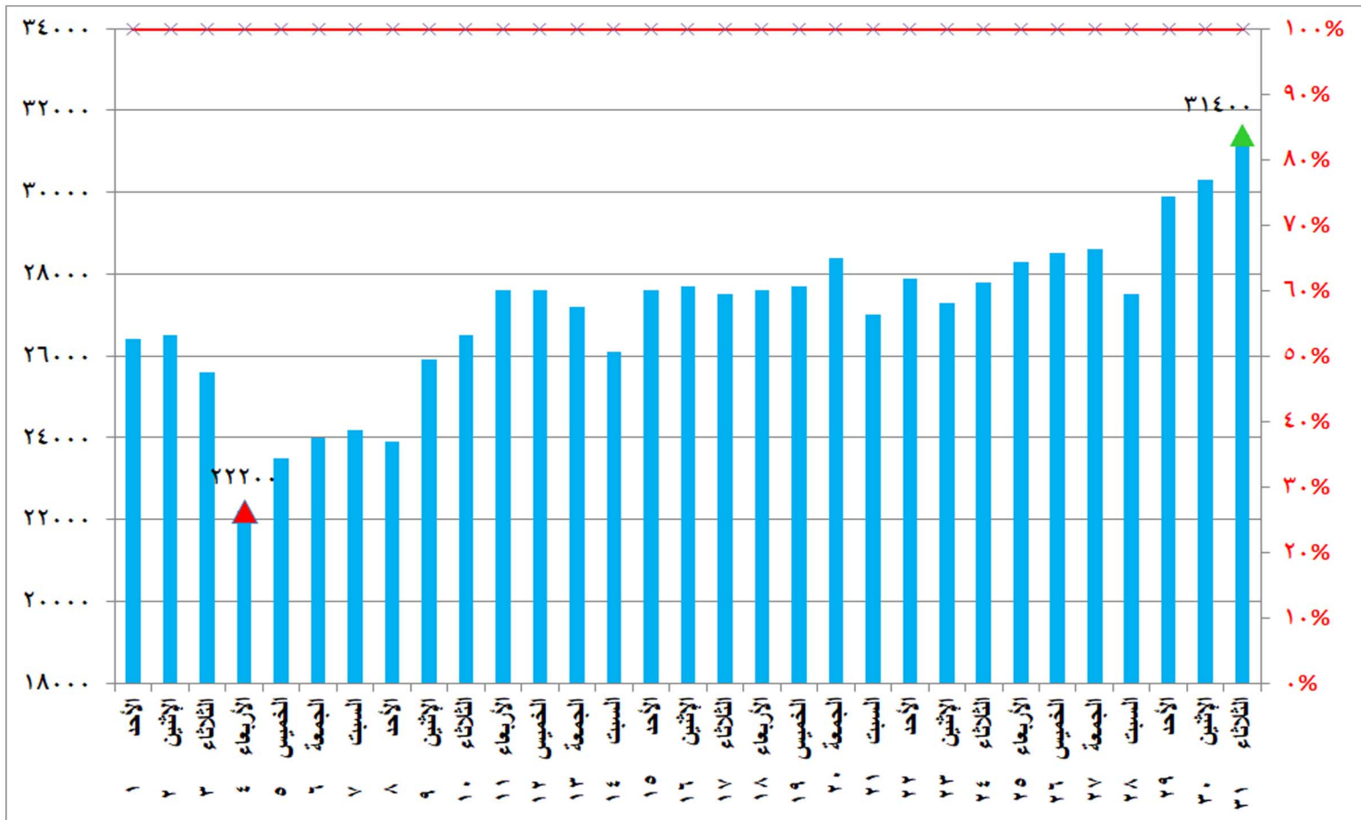
شكل (٥) قدرات الانتاج المتاحة ونسبتها للحمل الأقصى خلال شهر مايو ٢٠٢٢
