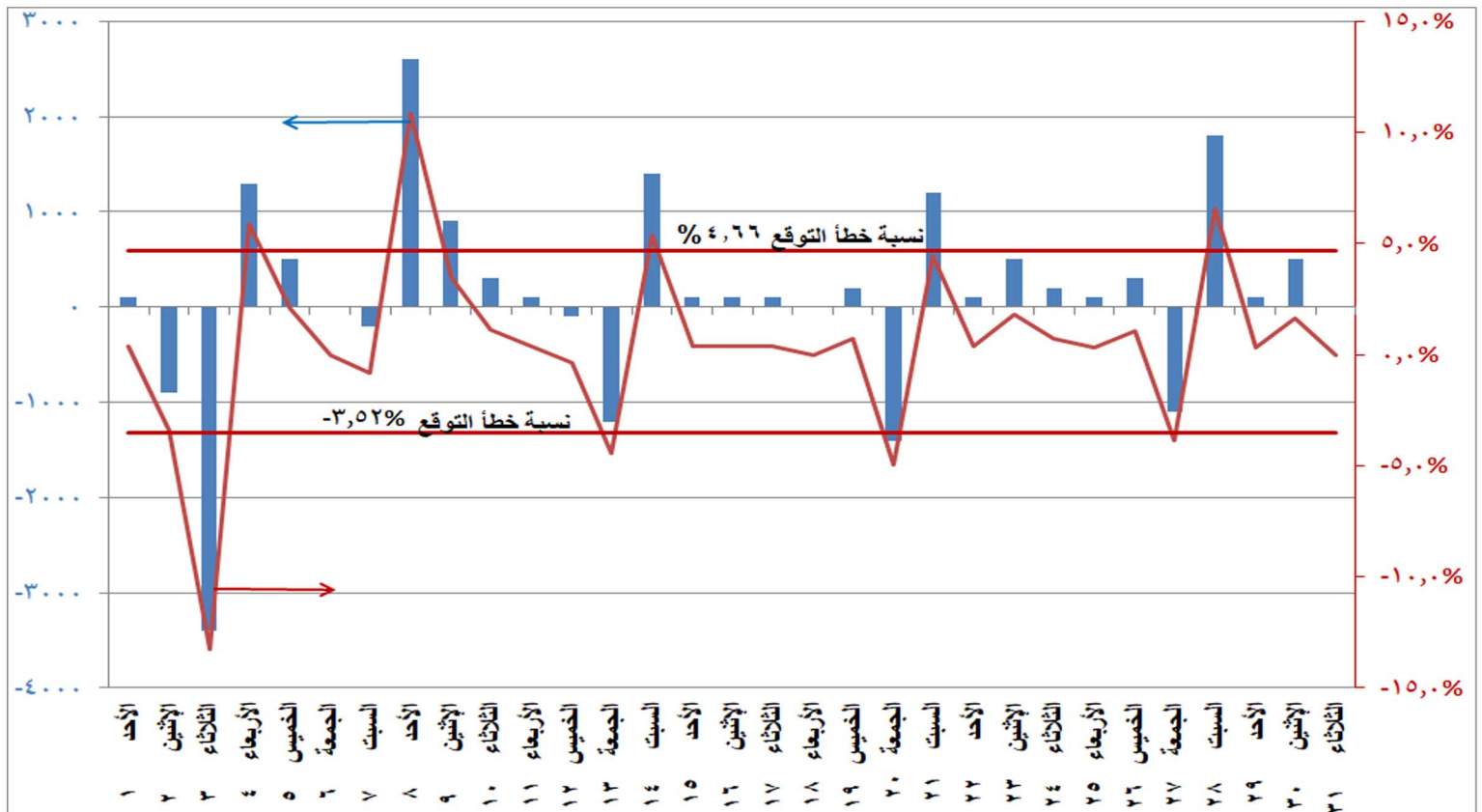
شكل (١٠) الفرق بين الحمل الأقصى المتوقع والمسجل فعليا ونسبة الفرق إلى الحمل المسجل فعليا خلال شهر مايو ٢٠٢٢
