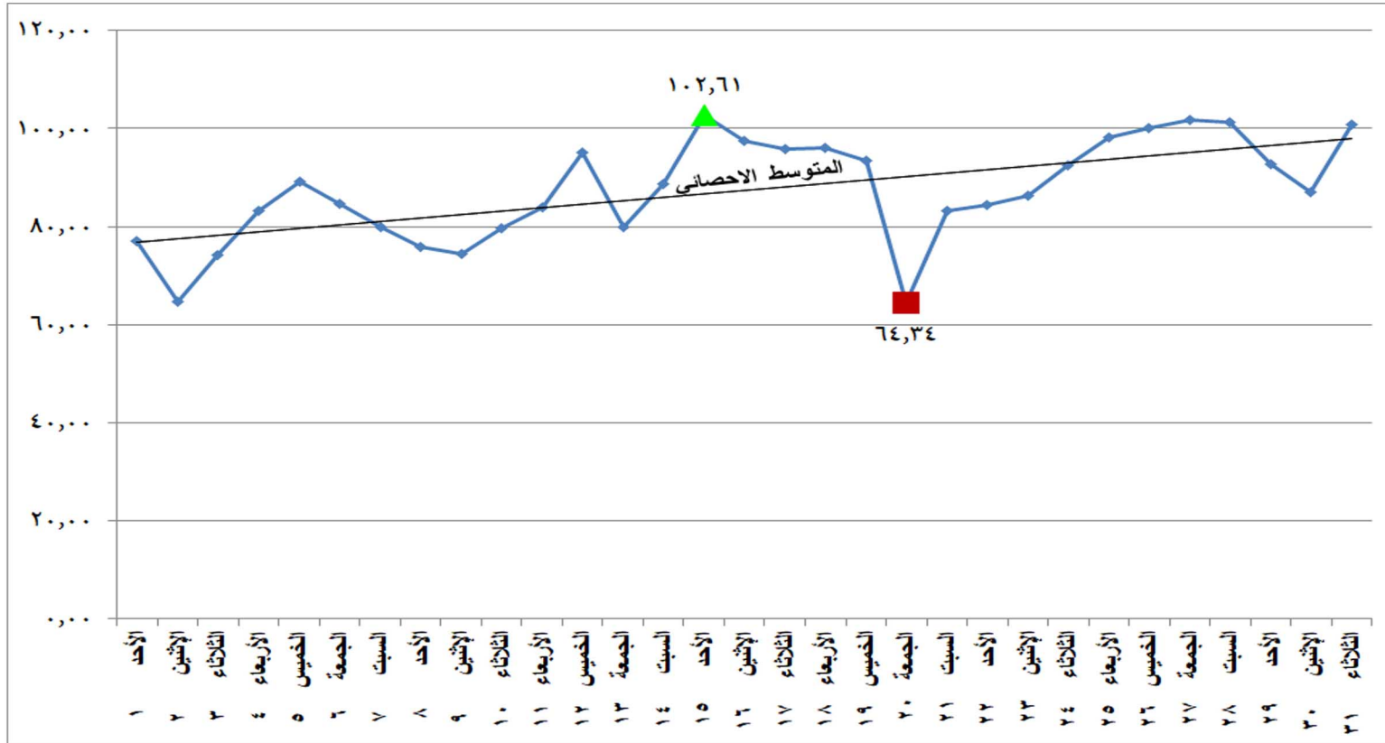
شكل (٢١) الطاقة الكهربائية المنتجة من المصادر غير الحرارية خلال شهر مايو ٢٠٢٢
