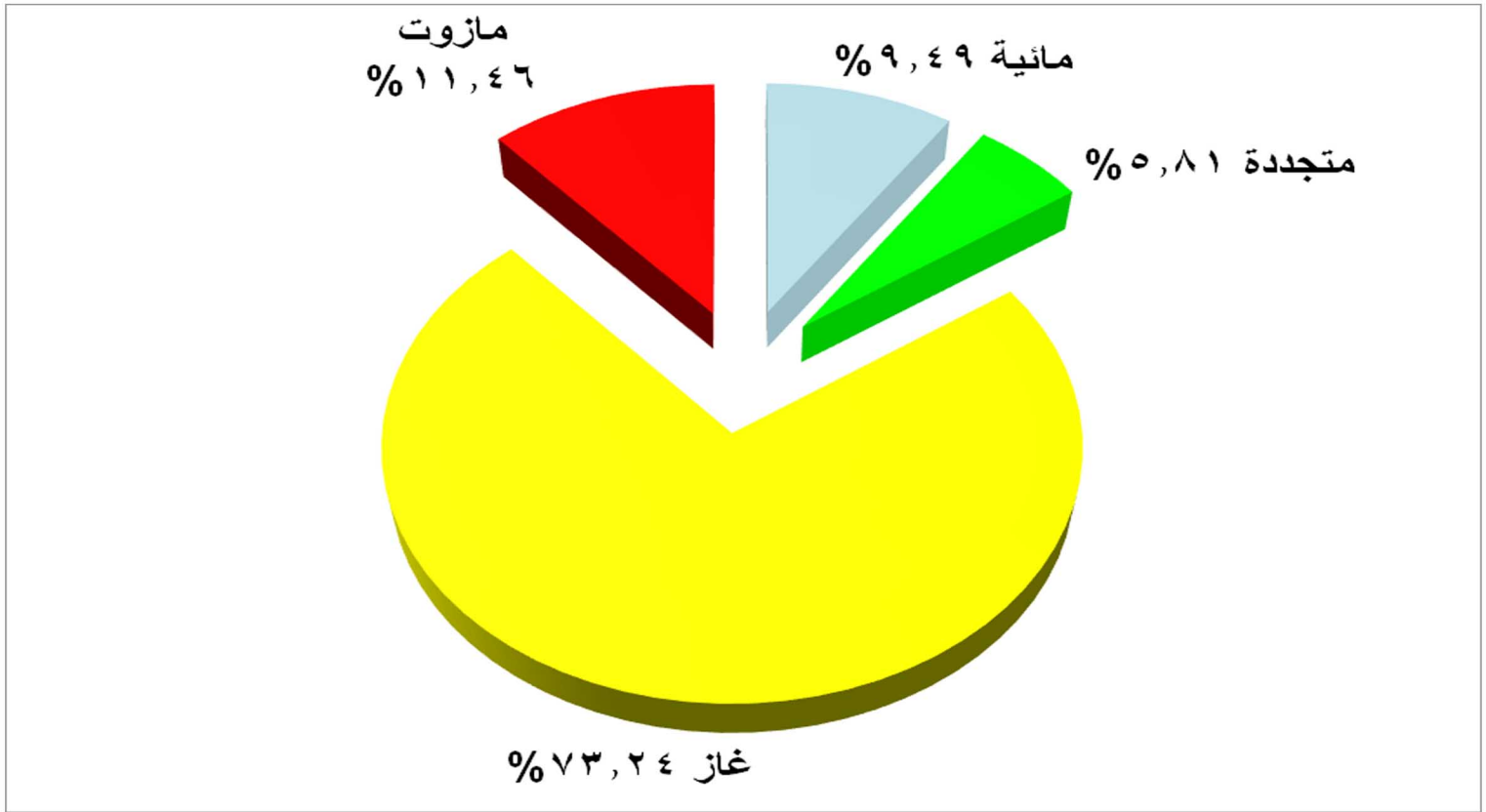
شكل (١٣) متوسط نسب مشاركة مصادر الطاقة الاولية في انتاج الكهرباء خلال شهر مايو ٢٠٢٢
