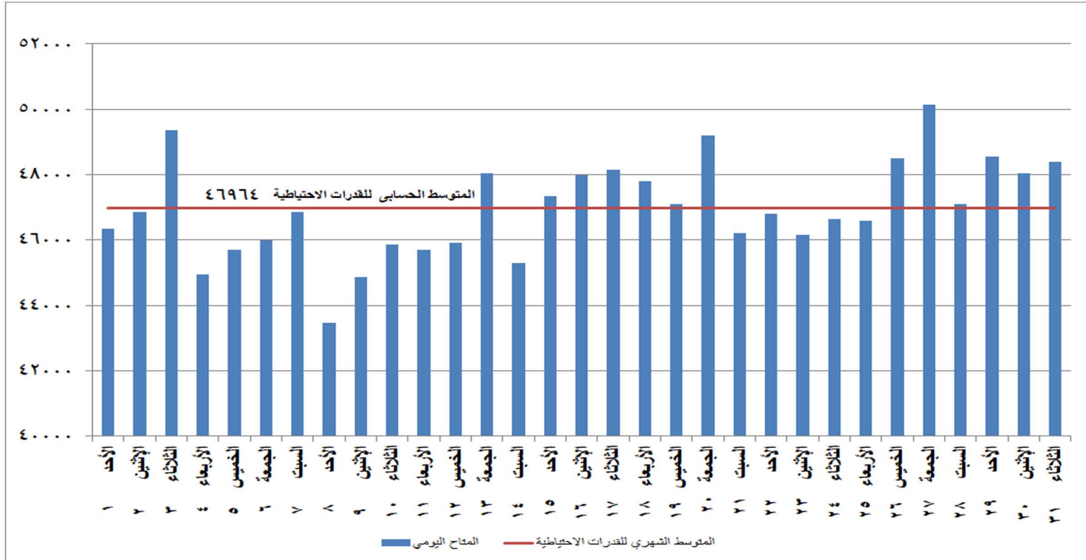
شكل (٢٧) القدرات المتاحة يوميا والمتوسط الشهري للقدرة الاحتياطية خلال شهر مايو ٢٠٢٢
