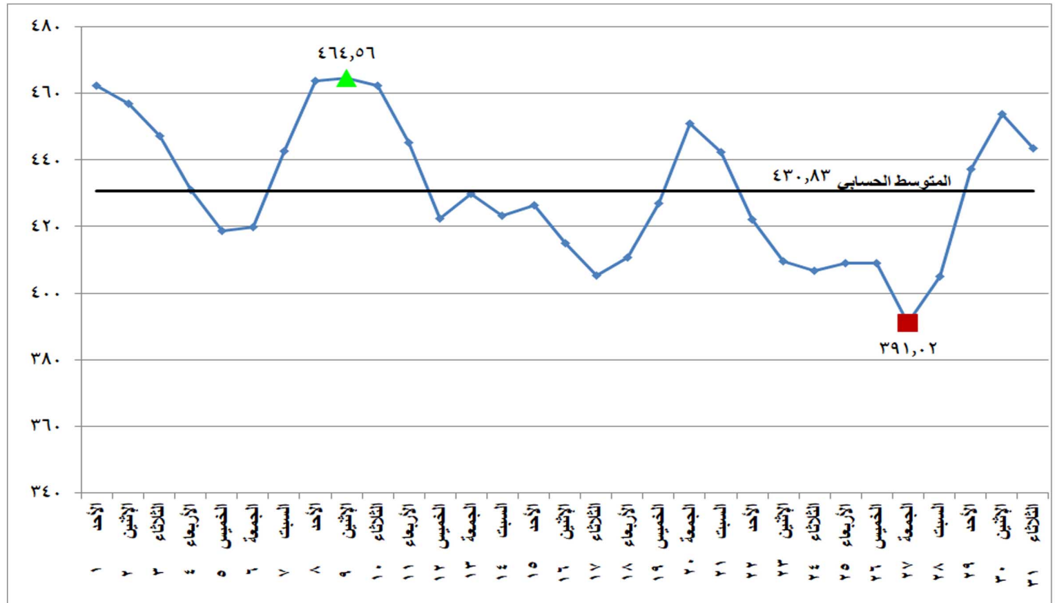
شكل (١٤) معامل انبعاثات غاز ثاني اكسيد الكربون المكافئ على مدى شهر مايو ٢٠٢٢
