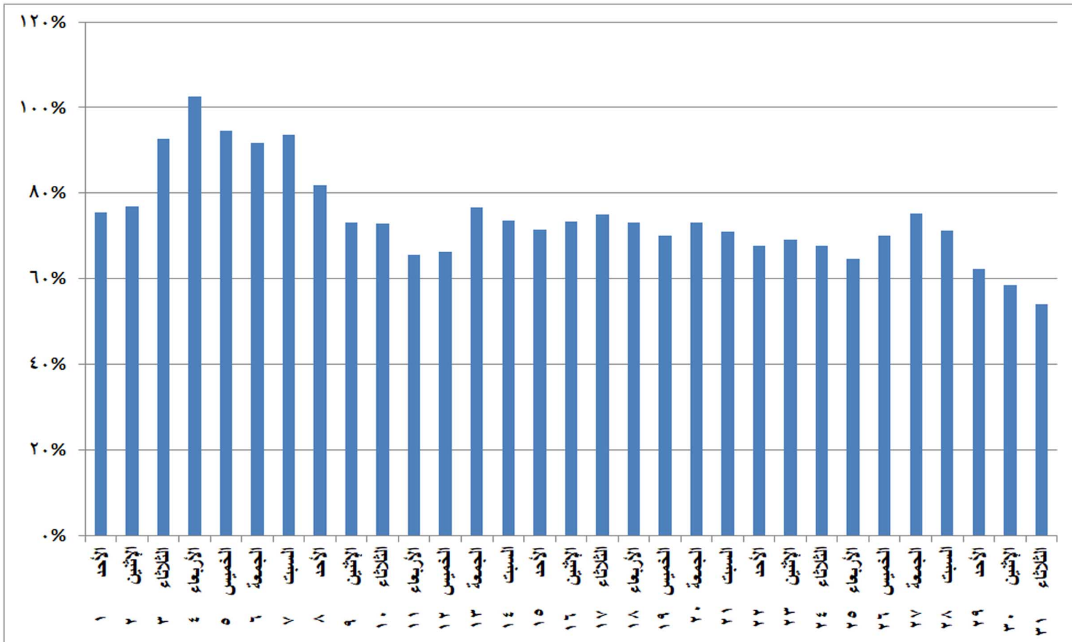
شكل (٢٨) نسب الفائض للحمل الاقصى المسجل يوميا خلال شهر مايو ٢٠٢٢
